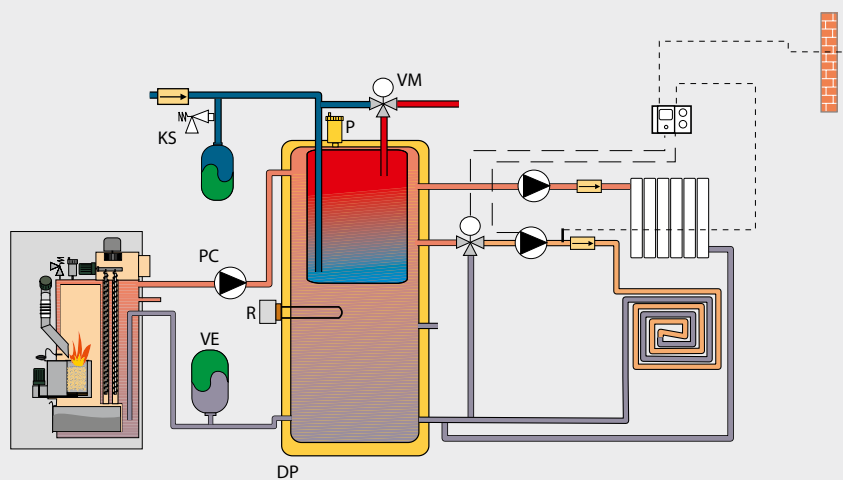
ESQUEMA DE PRINCIPIO BT DUO
