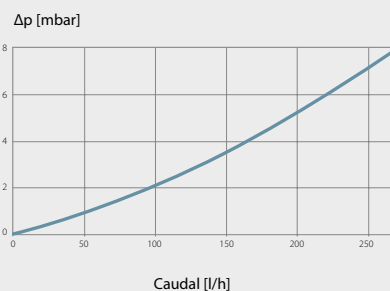
CURVA DE PERDIDA DE CARGA
